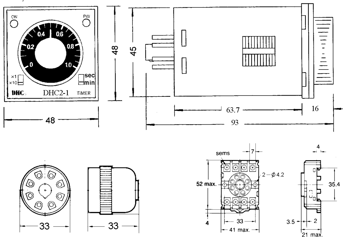
面板式插座
